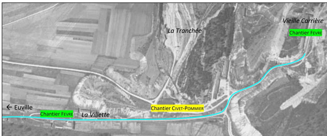
L'itinéraire de la voie entre la Vieille Carrière et le chantier de taille du Chemin de La Villette.
